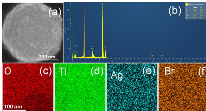
Fig. S2 SEM and EMIs of Ag-AgBr@TiO 2 NPAS
