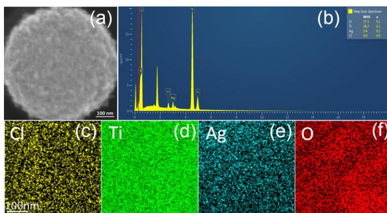
Fig. S1 SEM and EMIs of Ag-AgCl@TiO 2 NPAS
