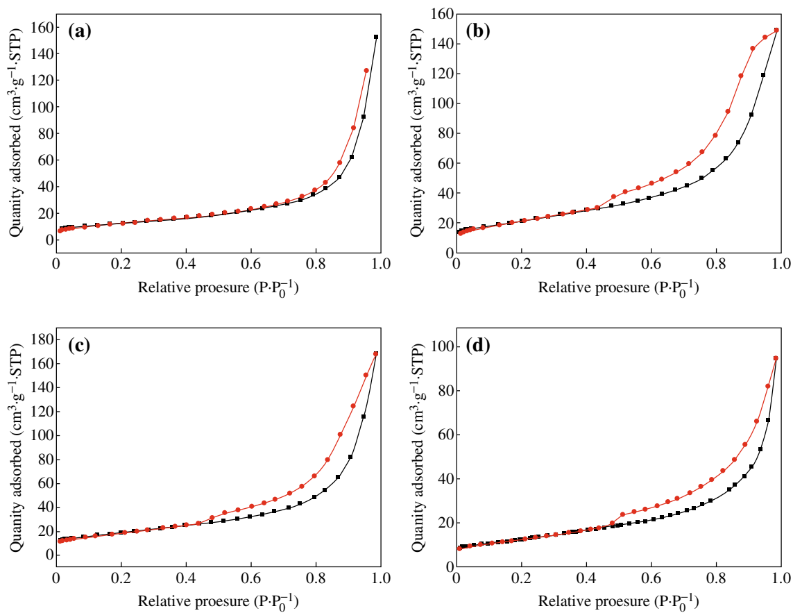
Fig. 3 Nitrogen adsorption/desorption isotherms of \text{CoFe}_2\text{O}_4 (a), \text{CoFe}_2\text{O}_4 -GNSs (b), \text{CoFe}_2\text{O}_4 -GNSs-350 (c), and \text{CoFe}_2\text{O}_4 -GNSs-550 (d)
